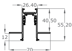
trimless recessed cod.: TK4820iTB L. 2 mt
